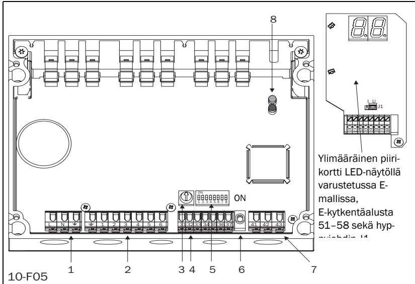
Fig. 4 Kytkentäalustojen jne. sijainti.
