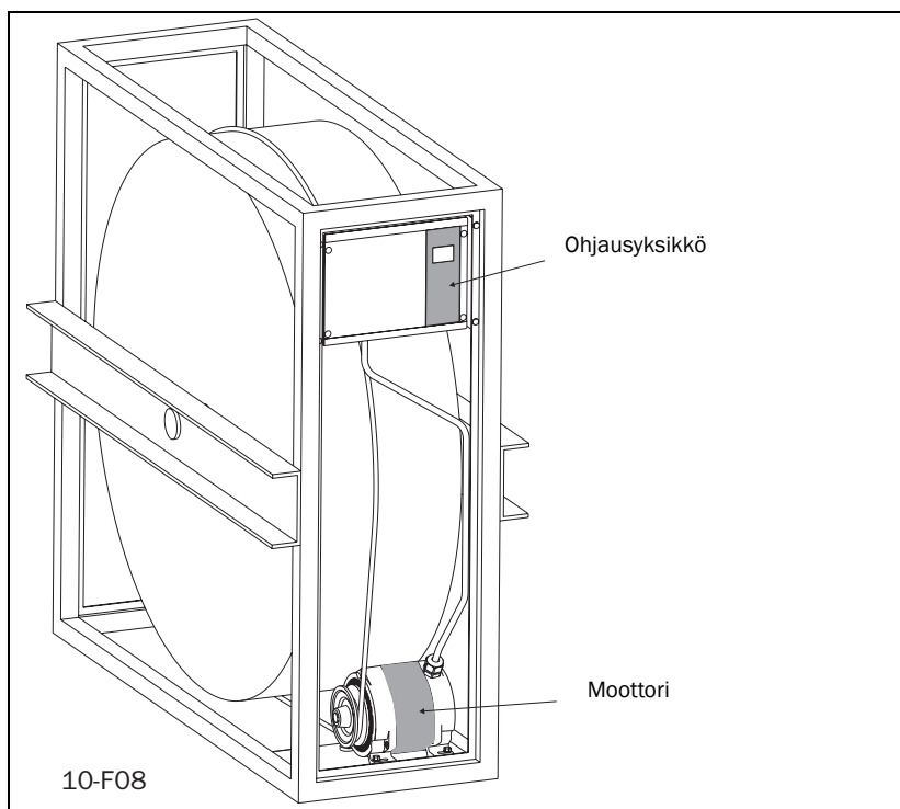
Fig. 1 Käyttölaitteella varustettu roottori.
