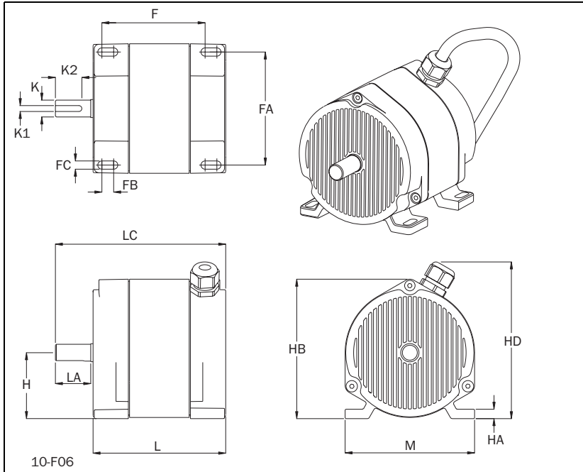
Kuva 6 Mitat, moottori.
